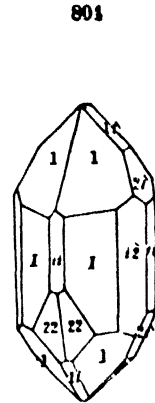
Crocoite.
